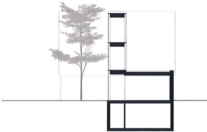
COUPE BB TRANSVERSALE
