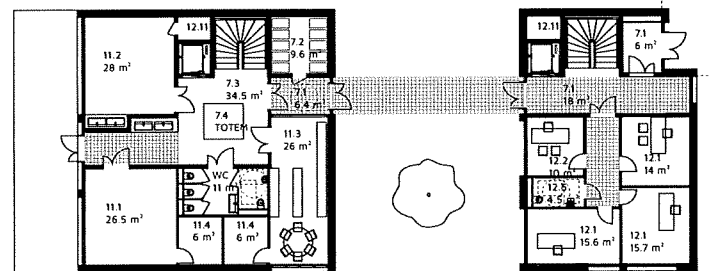
REZ-DE-CHAUSSEE
