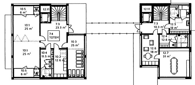
ETAGE 1
