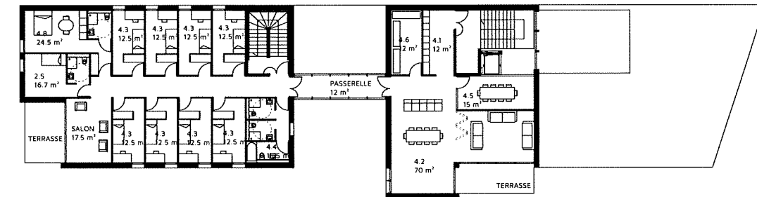
ETAGE 1
