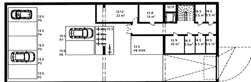
SOUS-SOL
