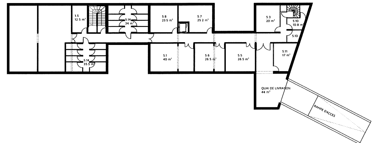
SOUS-SOL
