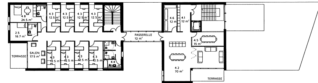
ETAGE 2
